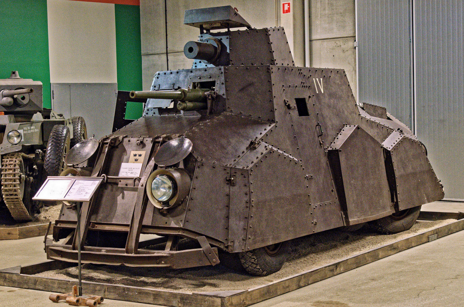
Pansarbil FM 29
